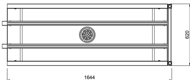
Boven aanzicht
