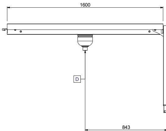
Zij aanzicht
